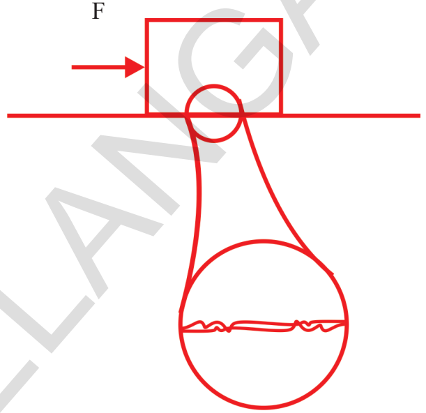
ಚಿತ್ರ - 10 ಎರಡು ಸಮತಳದಲ್ಲಿರುವ ಕ್ರಮರಹಿತ (ಅಕ್ರಮ) ಸ್ಥಿತಿ.
